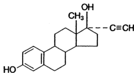
ETHINYL ESTRADIOL
